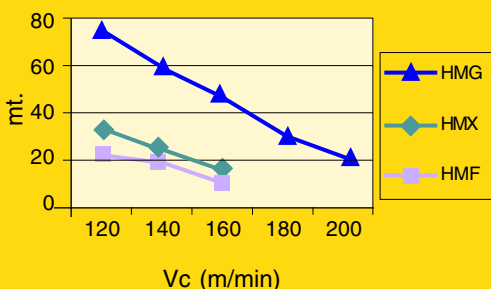
Risultati ottenuti su materiale DIN 1.2714
