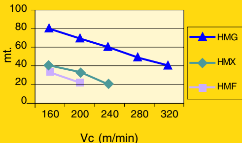
Risultati ottenuti su materiale C45 bonificato
